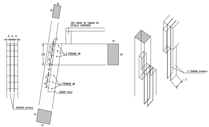
Figura 5a y 5b. Unión semirrígida de las vigas de piso.
