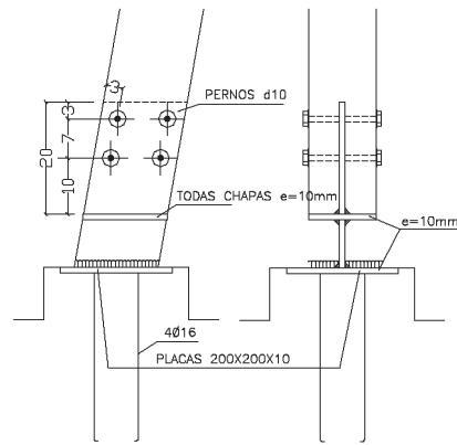
Figura 4a y 4b. Contacto con la solera mediante pieza metálica.
