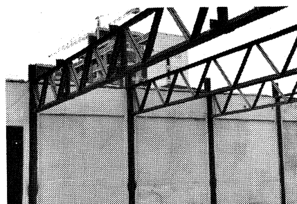
Unión viga-pared.
