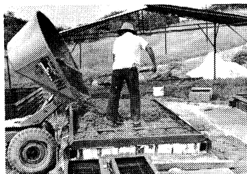
Vaciado de elemento prefabricado.
