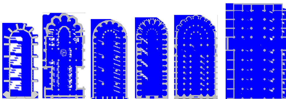
Figura 4. Expresividad de las muestras. De Izquierda a derecha: Sainte Chapelle y León (Muy expresivas), Sta. María y Gerona (Expresivas) y Toledo y Sevilla (Mudas). Medidas según recreación informática para el día 21 de junio del año 1600 a las 12:00 horas. Autor: Juan M. Medina.
