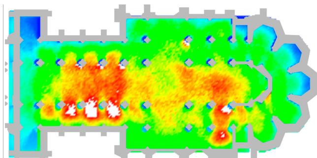
Figura 3. Reflejo de la intensidad en la Catedral de León el 21 de Marzo a las 12:00 según proyecto original. Autor: Juan M. Medina.
