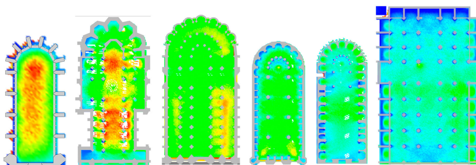
Figura 5. Intensidad de iluminación de las muestras. De Izquierda a derecha: Sainte Chapelle y León (Intensidad alta); Toledo, Sta. María y Gerona (Intensidad media) y Sevilla (Intensidad baja). Medidas según recreación informática con 3ds Max Design 2011 para el día 21 de Junio del año 1600 a las 12:00 horas. Autor: Juan M. Medina.
