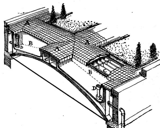
Fig. 47.—Bóveda para sostener un jardín: AA: Pasos (las pendientes para desagüe se han exagerado en el dibujo). BB: Bolsones para tierra vegetal. CC: Tabiquillos. DD: Desagües de los bolsones. Los taberos que forman los elementos A y B se apoyan sobre los tabiquillos, dejando libres los movimientos de dilatación. Los bolsones se enjoscán con mortero hidráulico.
