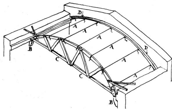
FIG. 3.—Preparación para construir una bóveda cilíndrica empleando cuerdas como guías. AAA: Cuerdas tensadas paralelas al eje del cilindro. BB : Egiones para apoyo de la cercha. CC : Cercha ligera en que se sujeta un cabo de cada cuerda. DD : Raza en el muro de testa, en cuyo borde inferior se sujeta el otro cabo de cada cuerda. El resto de la construcción, como en la figura 1; las cuerdas molestan algo el trabajo.
