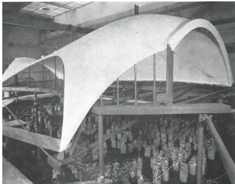
estructura laminar del Club Tachira Venezuela
