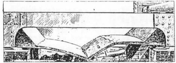
Figura 6.- Ensayo de colapso de una bóveda de hormigón armado Monier (Öst. Ing.- und Arch.- Verein 1895).
