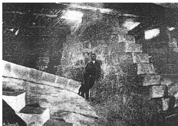
Figura 24.- Cargas sobre la clave central y los arcos transversales (Rubiò Bellver, 1912).
