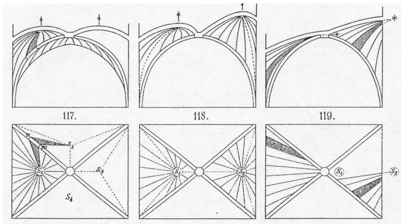
Figura 20.- Diferentes familias de cortes para el análisis de bóvedas góticas. (Ungewitter 1890)
