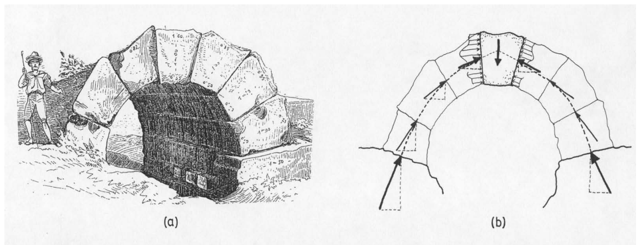
Figura 2.- Arco de dovelas etrusco. Estudio del equilibrio de las dovelas (Durm 1885).
