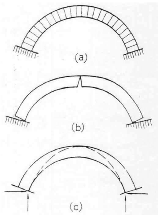
Figura 7.- Agrietamiento de un arco de fábrica tras el descimbrado (Heyman, 1995).
