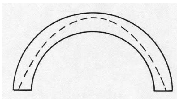
Figura 4.- Posible línea de empujes de un arco de medio punto (Heyman 1995).
