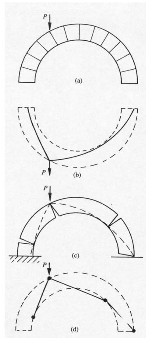
Figura 11.- Colapso de un arco de medio punto bajo una carga puntual. (Heyman, 1995).
