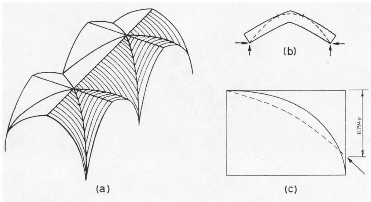
Figura 16.- Análisis límite de un bóveda gótica por el método de los cortes (Heyman, 1995).
