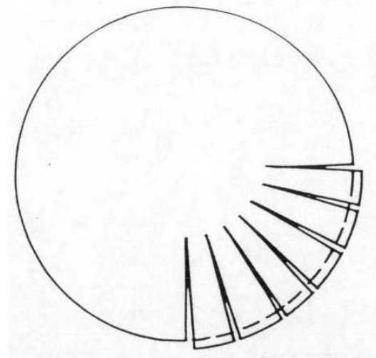
Figura 14.- Agrietamiento parcial de una cúpula (Heyman, 1988).
