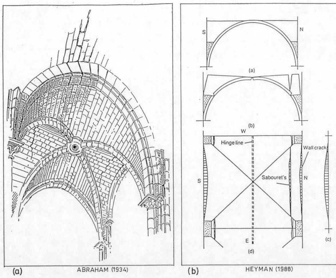
Figura 22.- Grietas en una bóveda gótica cutribartita. (Abraham, 1934).
