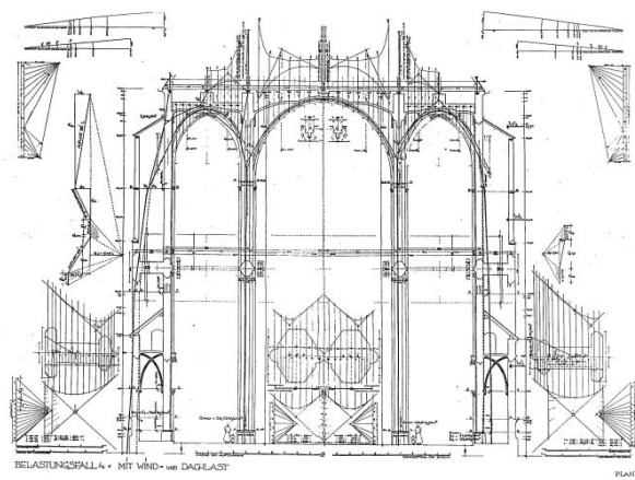
Figura 26.- Análisis del equilibrio de la iglesia de Sankt Martin en Landshut (Zorn, 1933).
