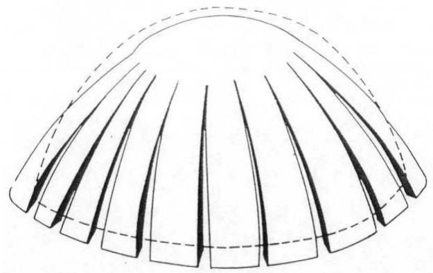
Figura 13.- Agrietamiento típico de una cúpula (Heyman, 1988).
