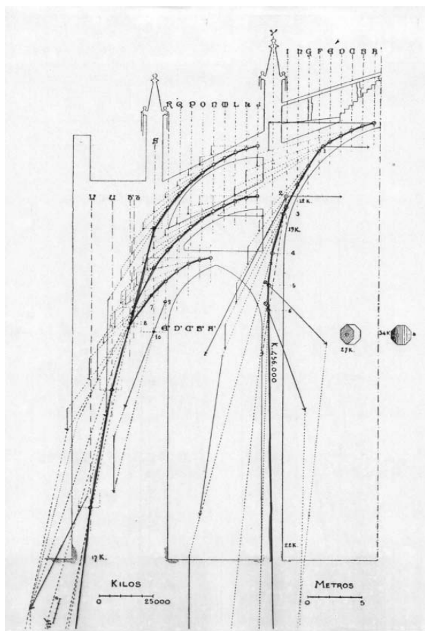
Figura 23.- Análisis del equilibrio de la catedral de Palma de Mallorca (Rubiò Bellver, 1912).
