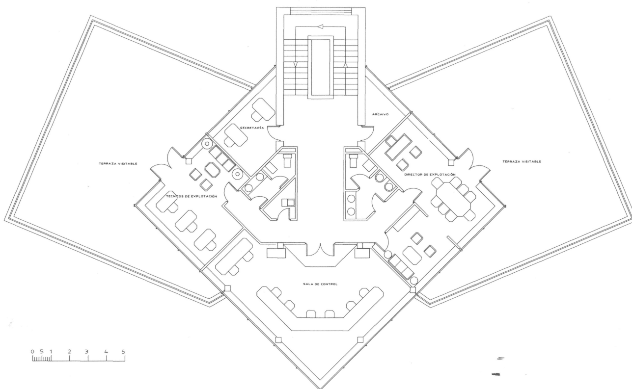
Planta primera.
